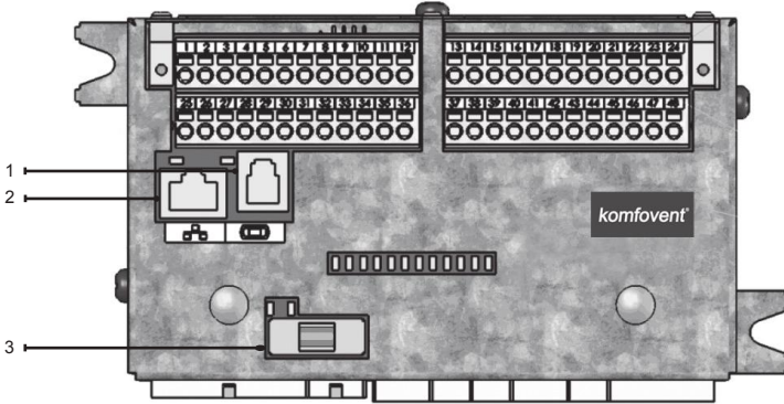
Rys. 1.3 a. Płyta główna
