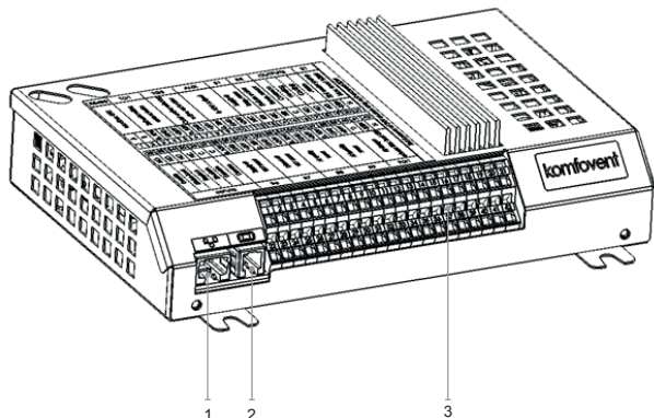
Rys. 1.3 a. Sterownik z zaciskami przyłączeń
